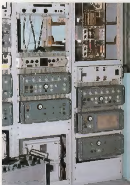
Kortegolfzender/ontvanger met antennetuner 1.5 - 29.999 MHz. 1955 1965.
